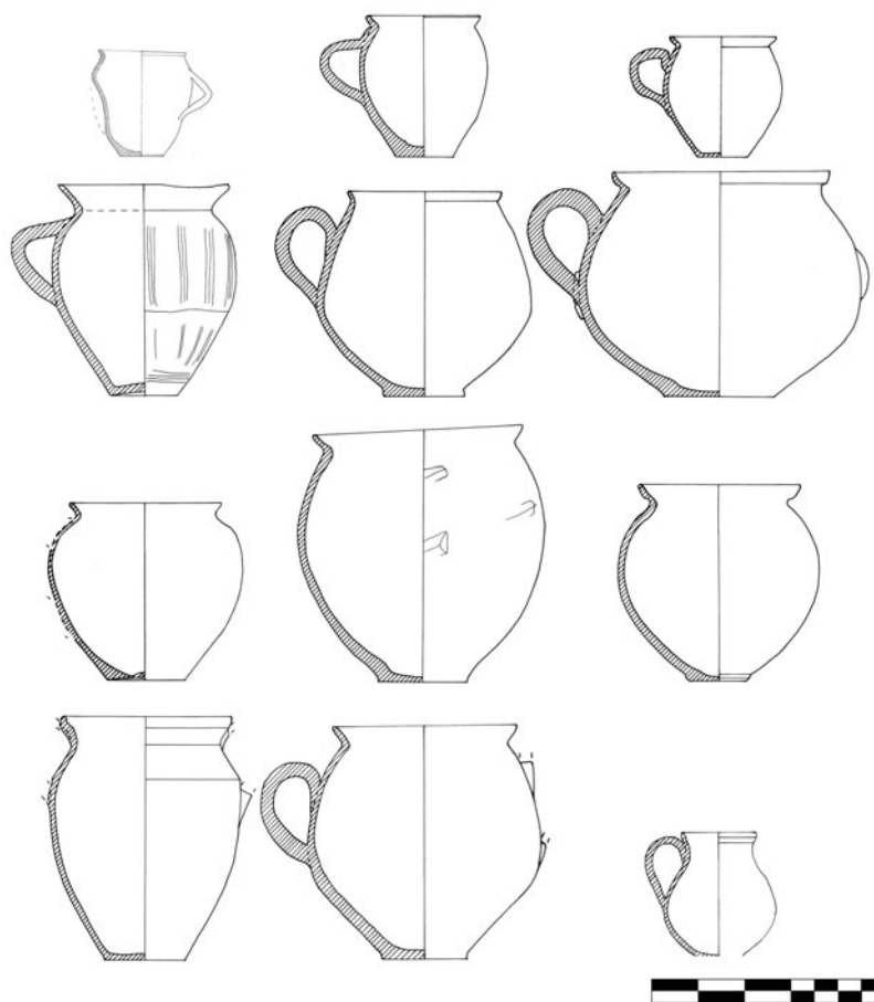
Fig. 2 Le tipologie di boccalini monoansati attestati (i disegni sono stati fatti da C. Ascarì Raccagni, G. Assenti, A. Gaucci)
